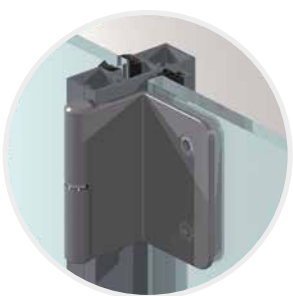
Detail PC1135™ 1 (idem PC1032™, PC1337™) Kozijndeel met scharnier
