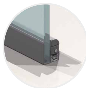
Detail PC1135™ 4 (idem PC1032™, PC1337™) Valdorpel onder volglazen geluidwerende deur
