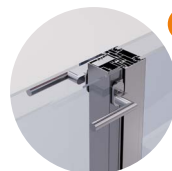
Detail PC4600F™ (idem PC4300F™, PC5000F™) Krukslot (of greep) met kozijndeel en geluiddichting
