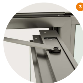
Detail PC4600F™ (idem PC4300F™, PC5000F™) Bovendetail kozijndeel met glasdeur en geluiddichting
